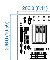
RCX-3430 PEG
